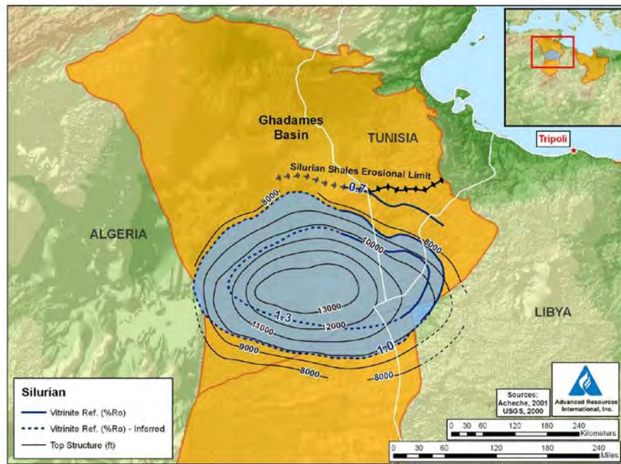
Figure VIII-4. Silurian Tannezuft Vitrinite Reflectance
