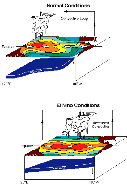
Normal vs. El Niño Conditions (Figure 6)
