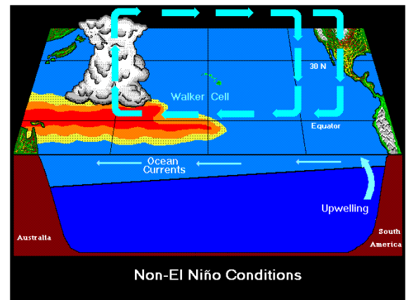
Non – El Niño Conditions (Figure 5)
