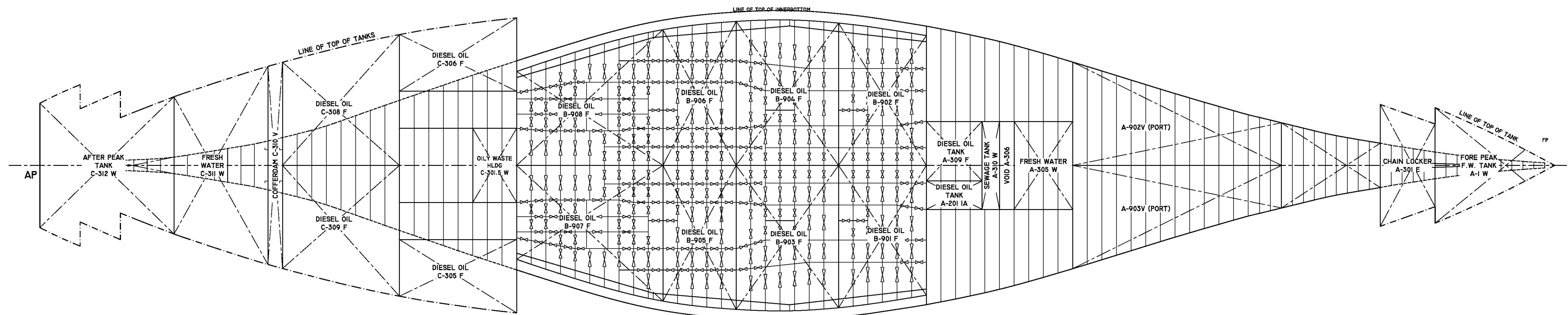
INNERBOTTOM
