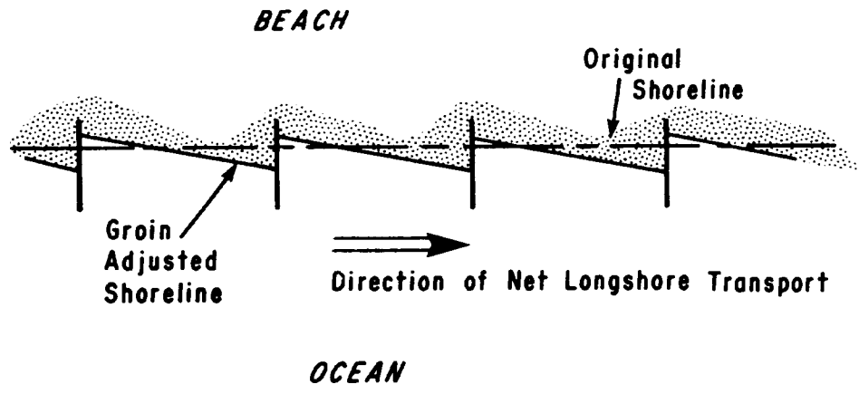
b. Multiple groins
