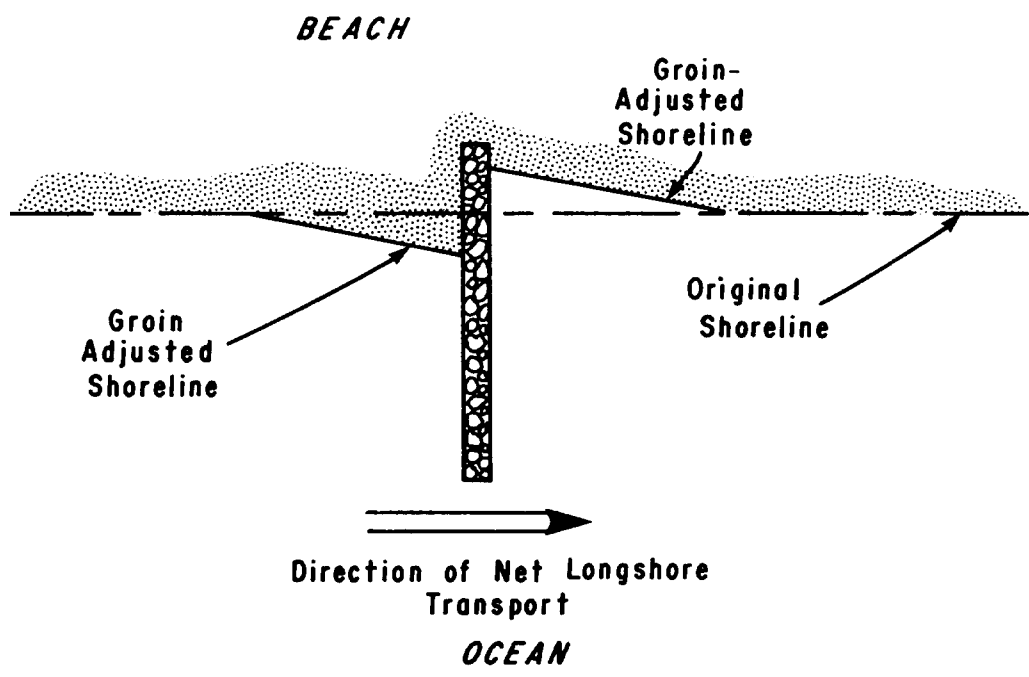
a. Single groin
