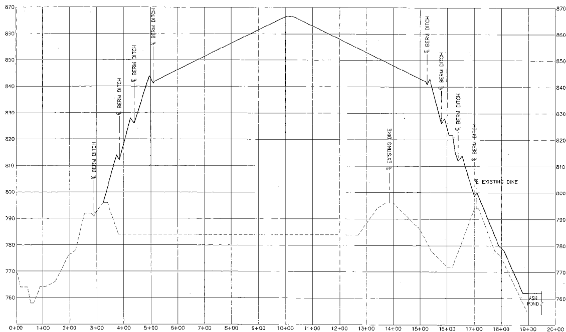
A17 - A17 1" = 100' HORIZ 1" = 10' VERT
