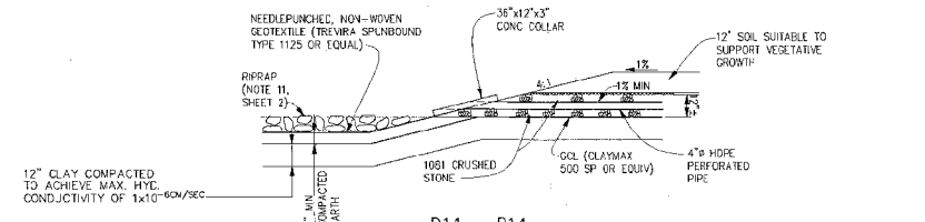
D14 - D14
