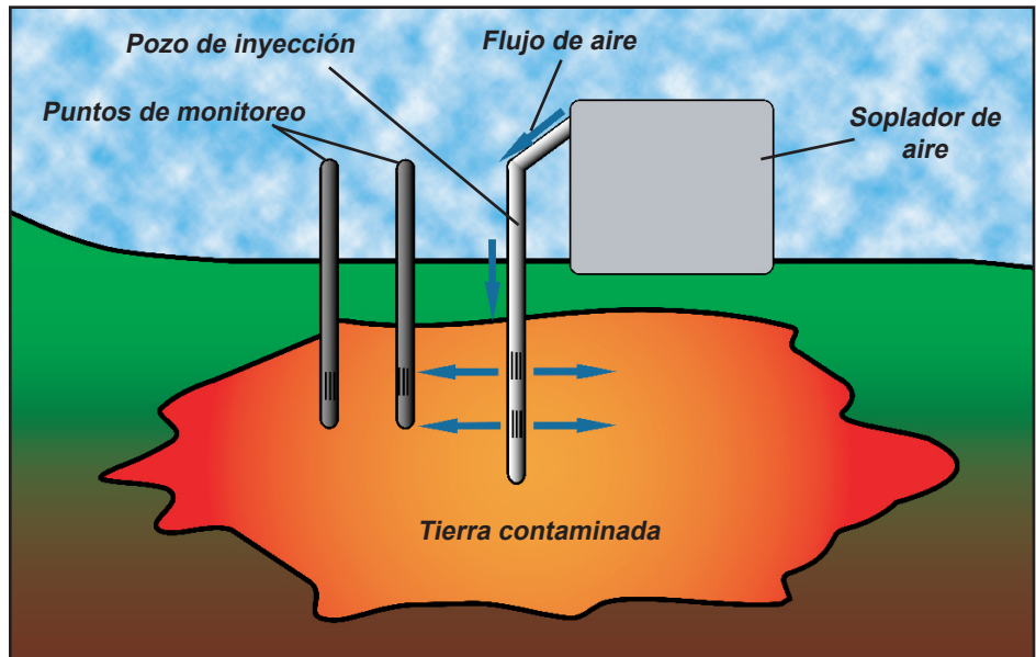
Un modelo del sistema de ventilación biológica.
