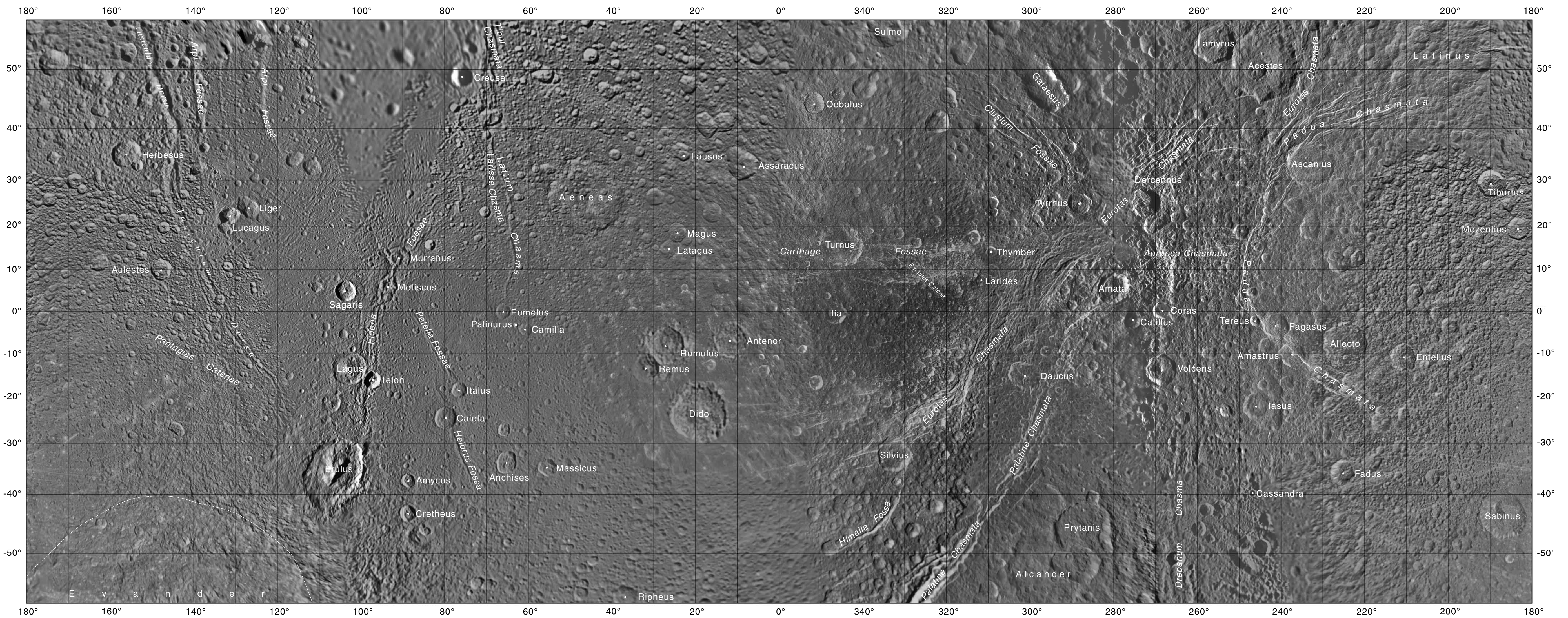
Dione
