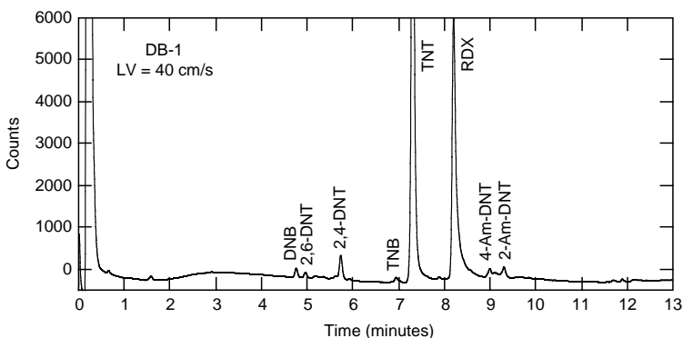
a. DB-1 analytical column.
