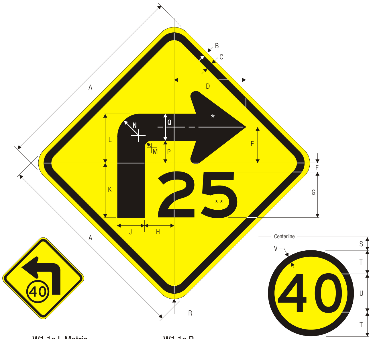
W1-1a L Metric
