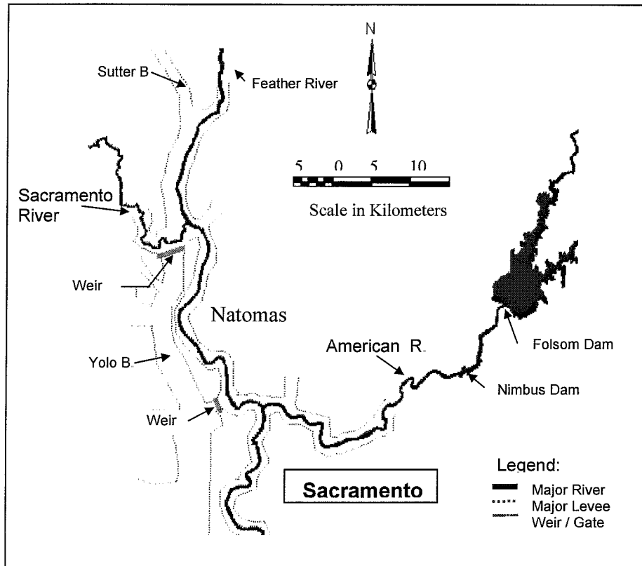
Fig. 2 Sacramento Area Flood Damage Reduction System Le système de maîtrise des crues les environs du Sacramento
