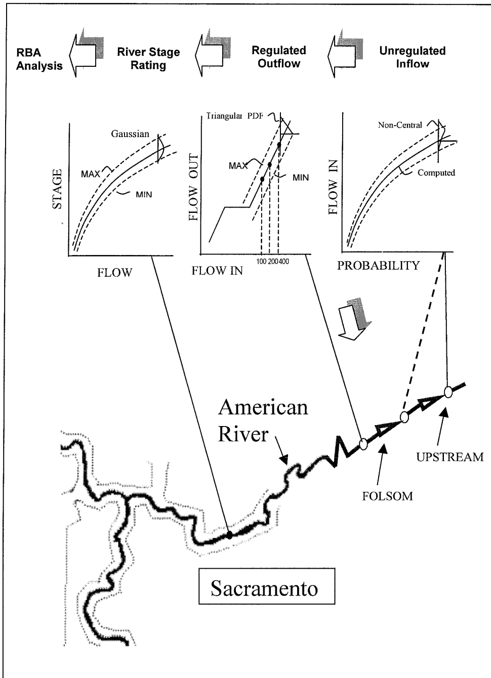
Fig. 3 Lower American River Hydrologic Uncertainty Analysis L'analyse de l'incertitude de la hydrologie du fleuve d'American
