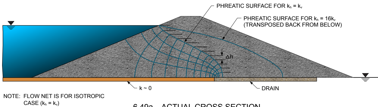
6.49a ACTUAL CROSS SECTION
