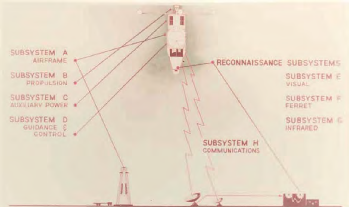
Fig. 1-4b — WS-117L Subsystems
