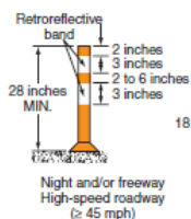
TUBULAR MARKERS
