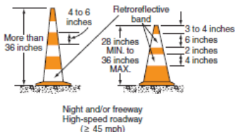
CONES
