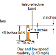
TUBULAR MARKERS
