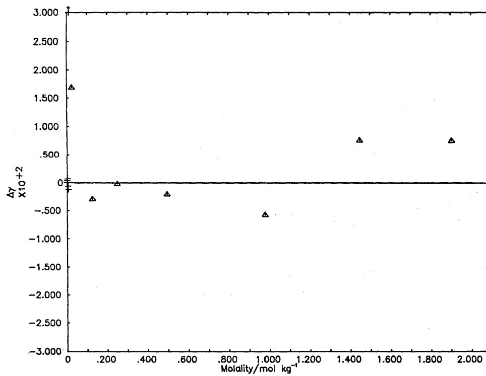
Deviation Plot for \text{Li}_2\text{SO}_4 : \Delta\gamma vs molality
