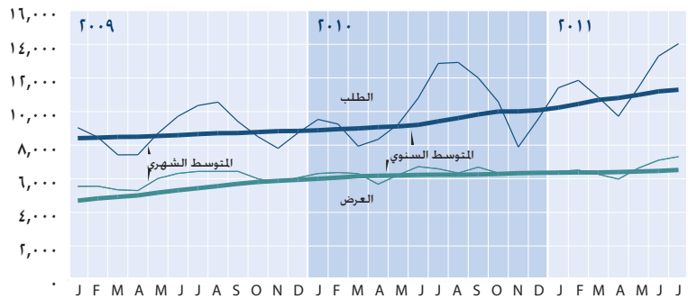
متوسط العرض من الكهرباء العراقية وتقديرات الطلب، حسب الشهر، ٢٠٠٩/٧-٢٠١١/٧ ميجاوات، على أساس المتوسط الشهري والسنوي
