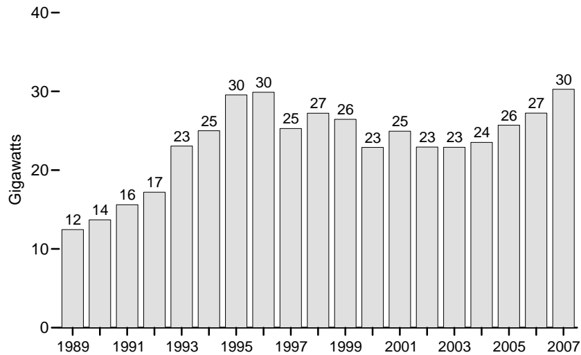
Actual Peakload Reductions Total, 1989-2007
