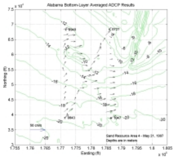
Bottom Layer
