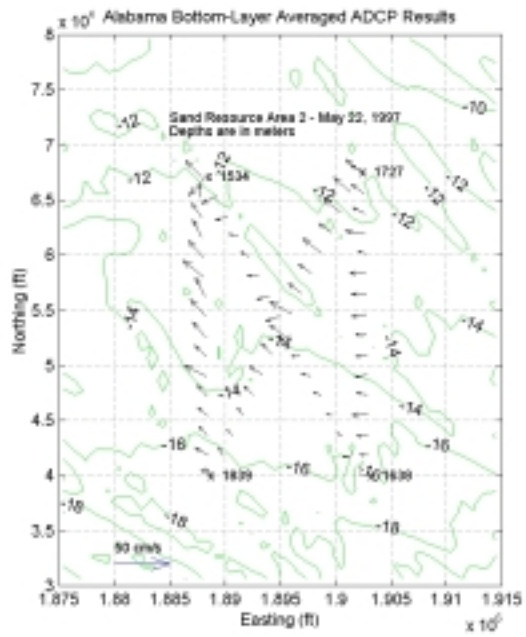
Bottom Layer
