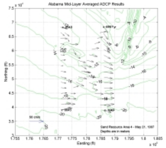
Middle Layer
