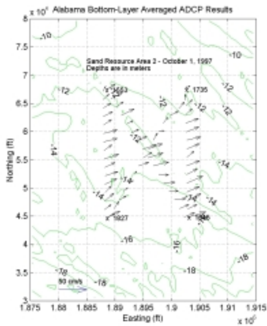
Bottom Layer
