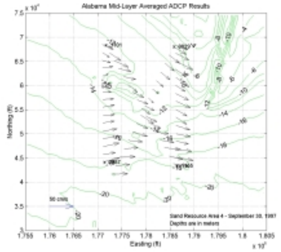
Middle Layer
