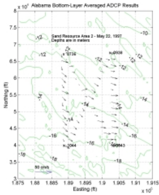
Bottom Layer
