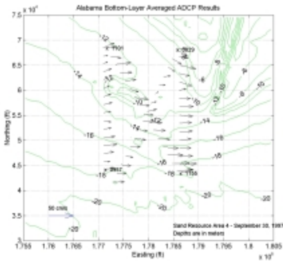
Bottom Layer
