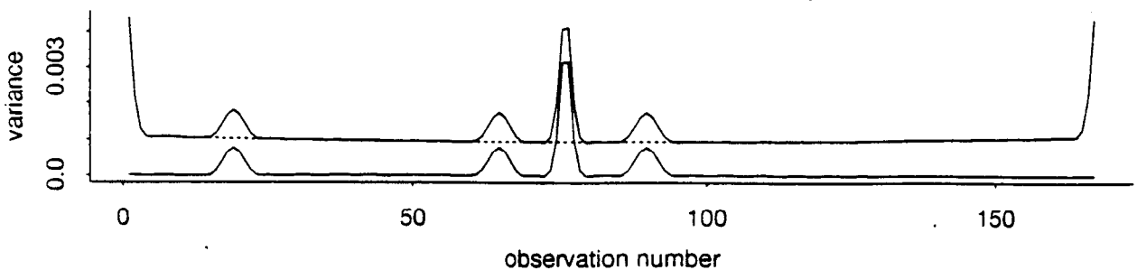
(d) variance of trend estimate
