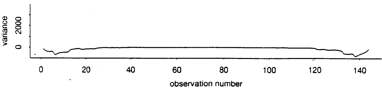
(d) contribution of covariances of e and (b 0 f)
