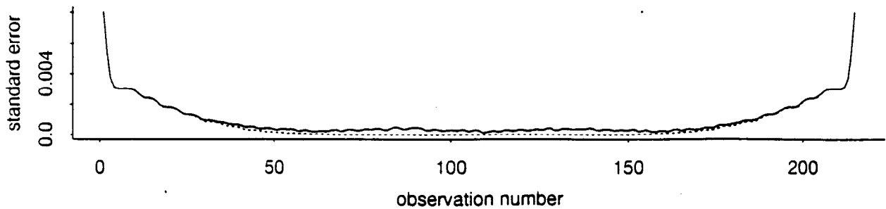
(d) standard error of trend estimate
