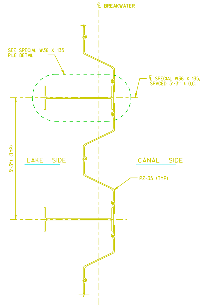
SECTION B SCALE: 1" = 1'-0"
