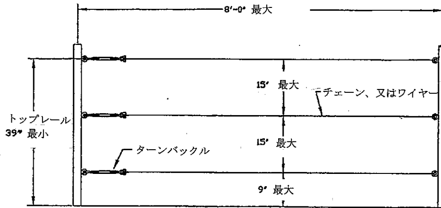
マリン、タイプB、3層式張力手摺
