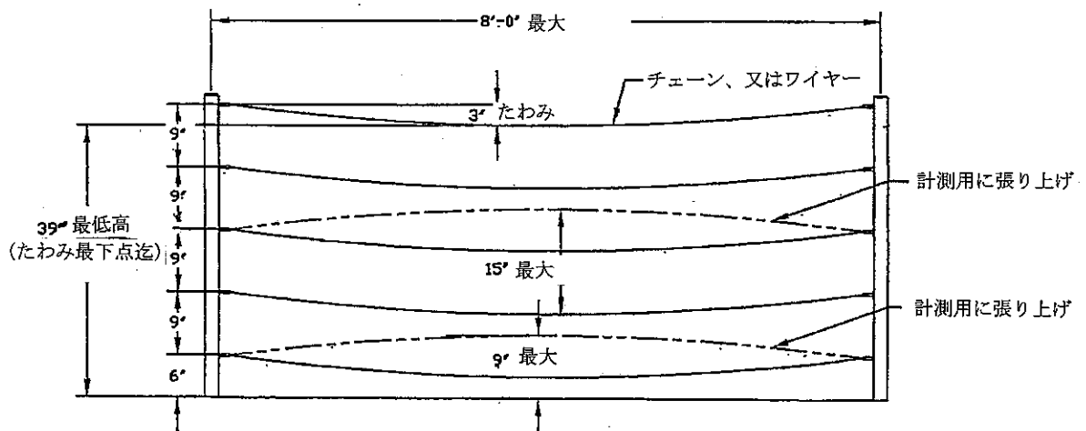
マリン、タイプC、非張力手摺 (3インチのたわみ)
