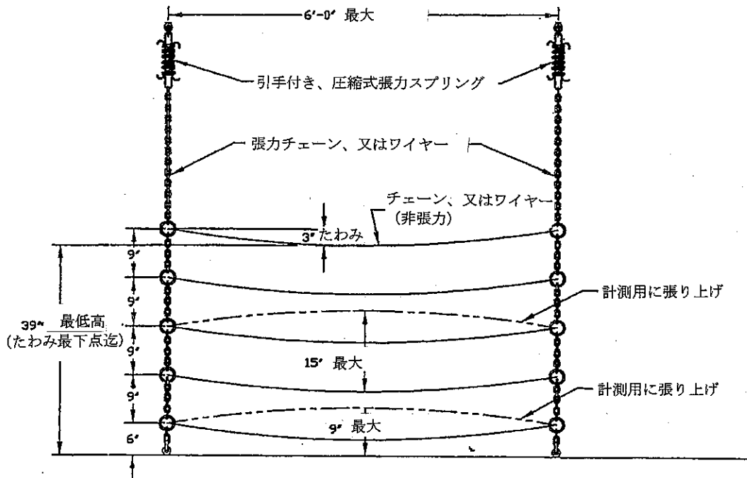
マリーン、タイプC、柔軟取り外し可能、 非張力手摺 (3インチのたわみ)
