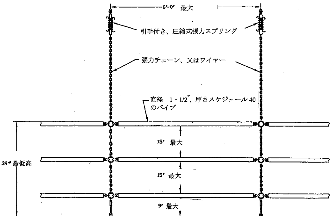
マリーン、タイプC、柔軟取り外し可能、 固定水平手摺
