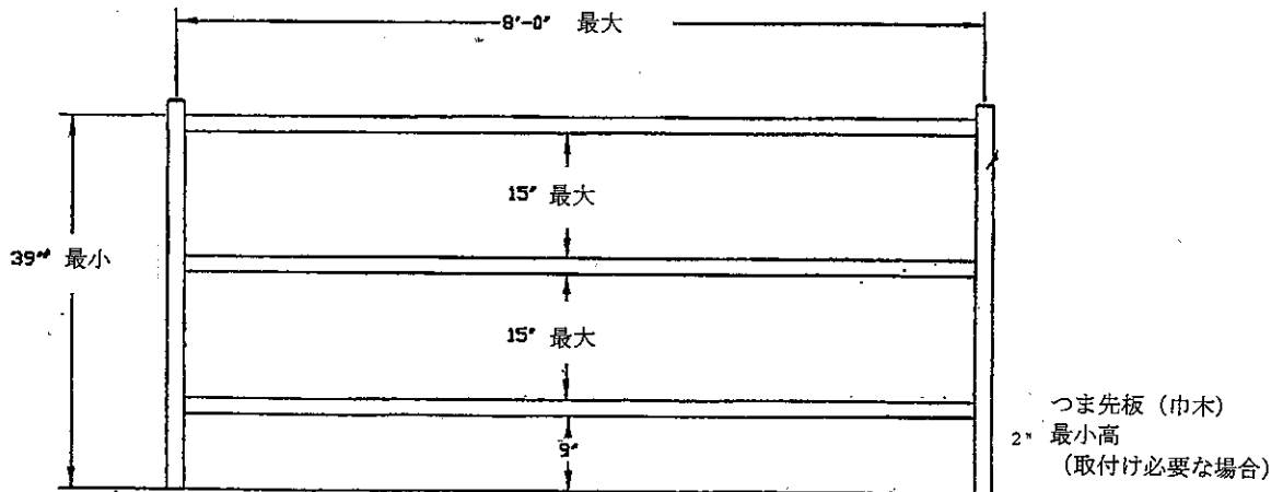
マリーン、タイプB、3層式固定手摺
