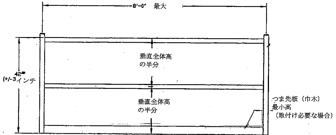
マリーン、タイプA、2層式固定落下防止手摺
