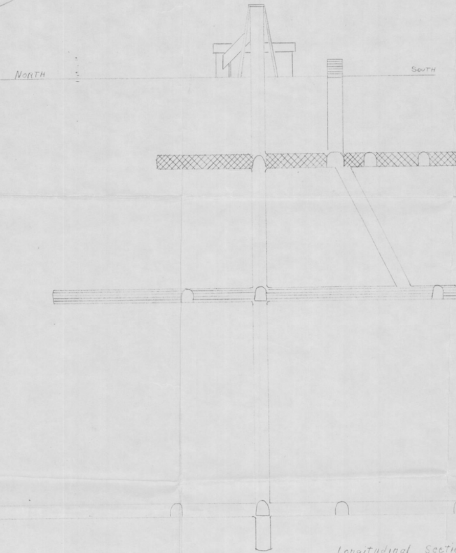
Longitudinal Section
