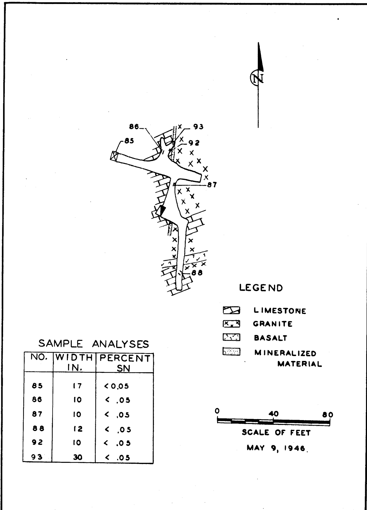
FIG. 6.- SUBLEVEL, BARTELL MINE, SEWARD PENINSULA.
