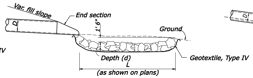
ELEVATION
