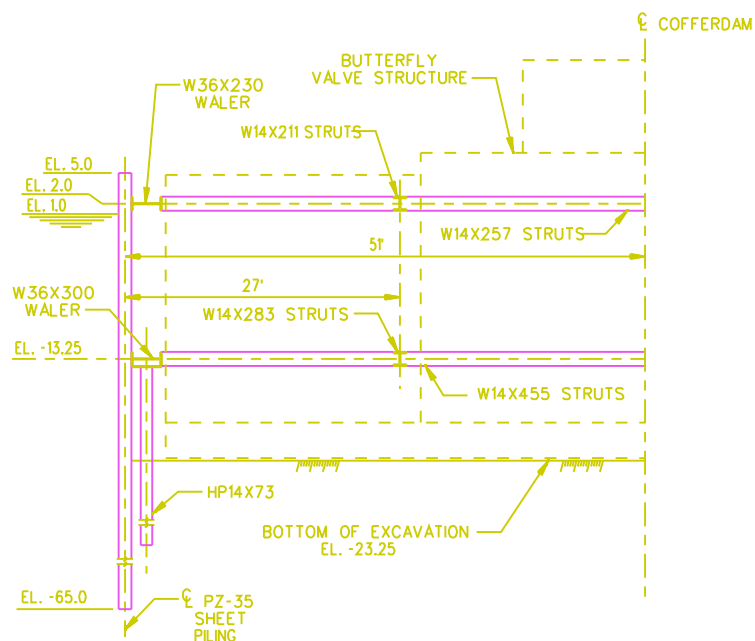
SECTION B 30 31 SCALE: 1/8" = 1'-0"
