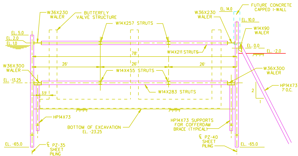
SECTION A 30 31 SCALE: 1/8" = 1'-0"
