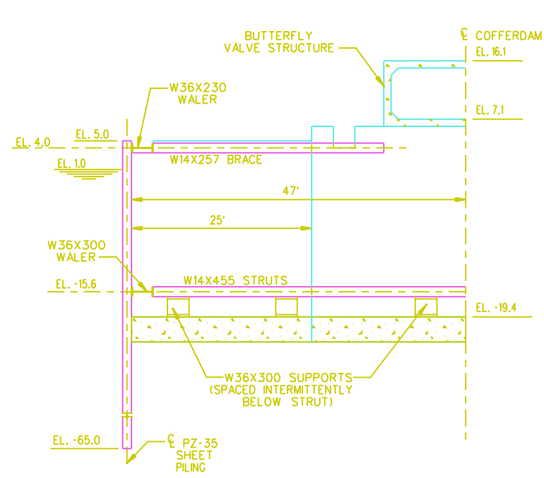
SECTION C 30 31 SCALE: 1/8" = 1'-0"
