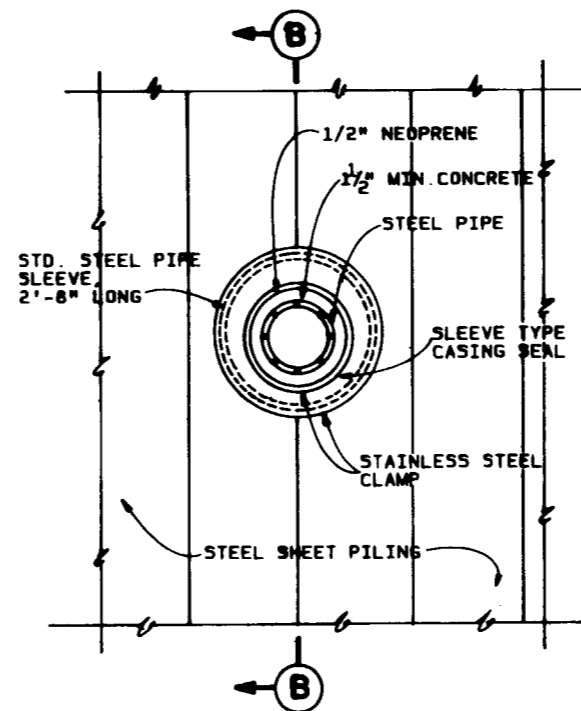
ELEVATION
