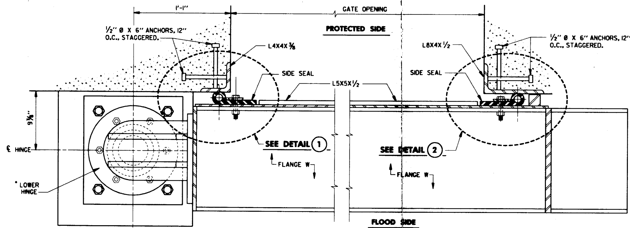
SECTION THRU SWING GATE SCALE: 3" = 1'-0"
