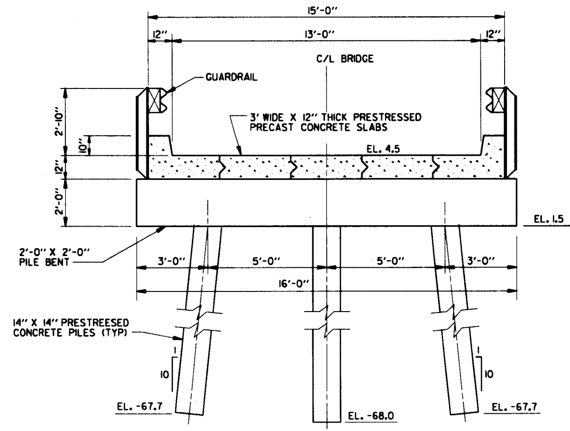
SECTION A SCALE: \frac{1}{2}'' = 1' - 0''
