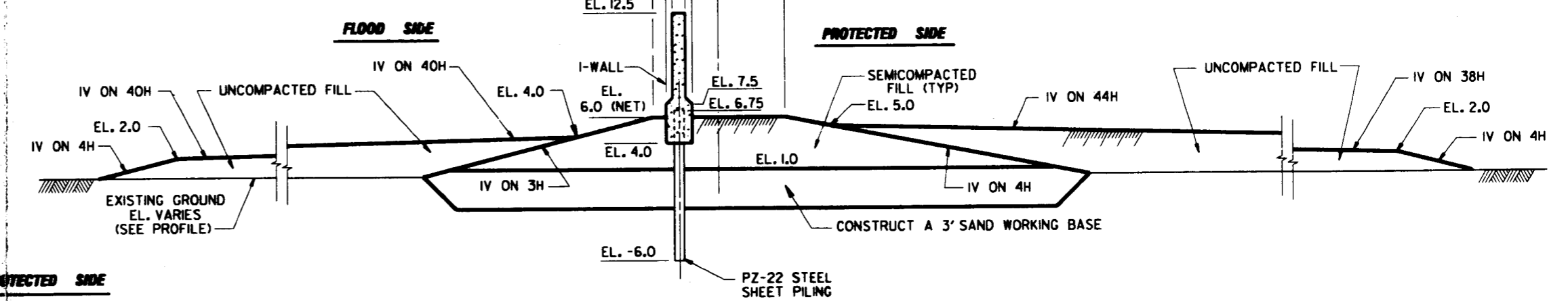
TYPICAL SECTIONS STA. 507+31 WL TO STA. 509+33 WL STA. 509+67 WL TO STA. 510+30 WL STA. 512+32 WL TO STA. 514+52 WL STA. 516+14 WL TO STA. 516+84 WL
