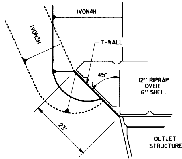
DETAIL 1 SCALE: 1" = 10'
