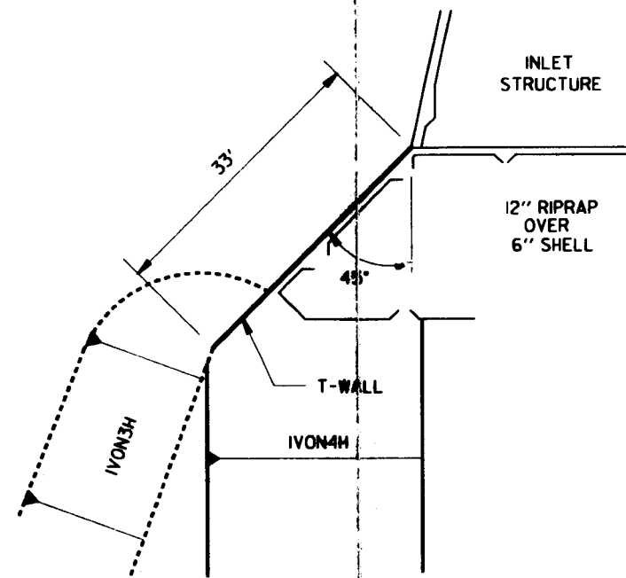
DETAIL 2 SCALE: 1" = 10'
