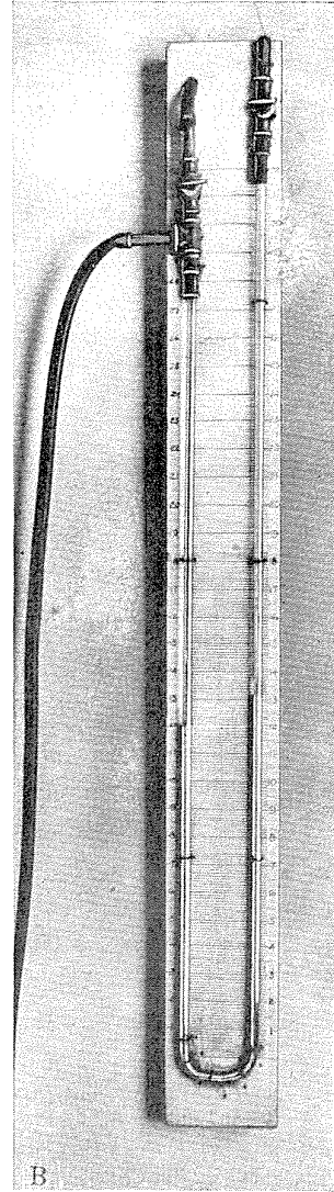
B, PIEZOMETER TUBE.
