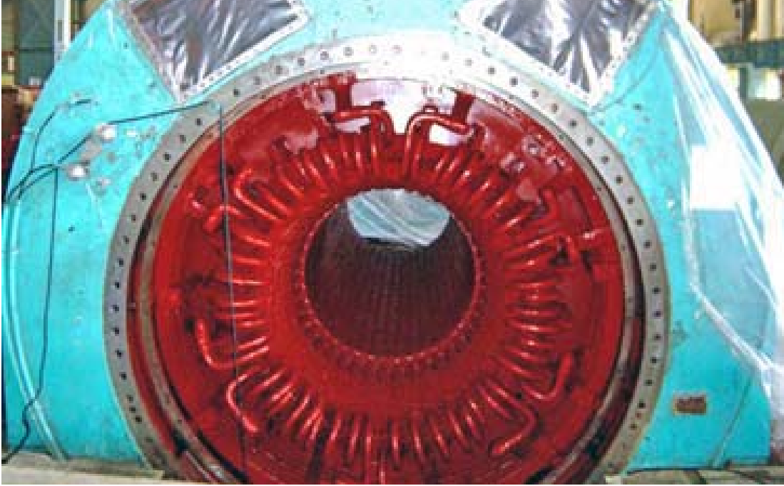
في الاعلى : مولد جديد وجهاز للفحص والتنصيب في احد اقسام انتاج الطاقة الكهربائية في جنوب العراق .
