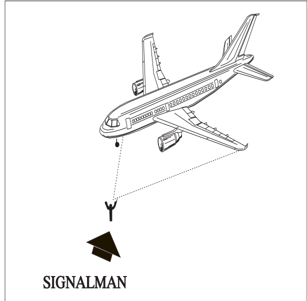
FIG 4-3-8 Signalman’s Position
