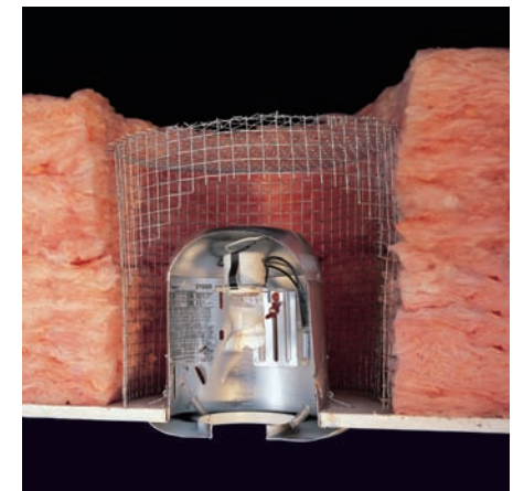
Use lámina metálica o malla metálica para crear una barrera alrededor de las lámparas o ventilación.
