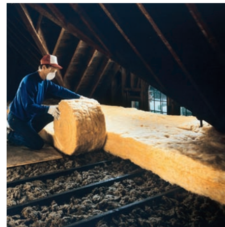
Coloque el rollo de aislamiento de fibra de vidrio perpendicular a las viguetas.
