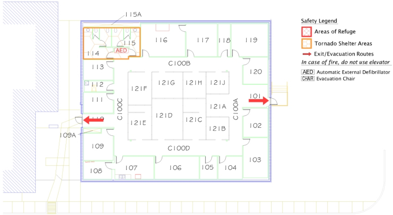
N FIRST FLOOR PLAN SCALE: N.T.S.
