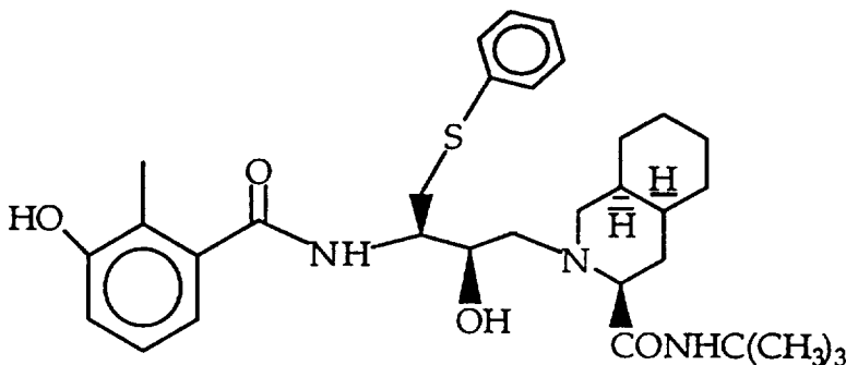
Nelfinavir Mesylate
