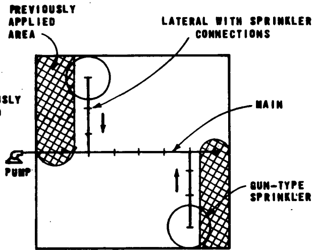
(d) STATIONARY GUN
