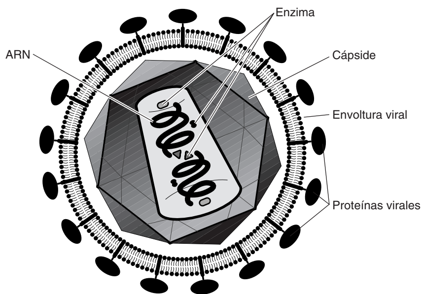
Estructura del Virus de Inmunodeficiencia Humana (VIH)
