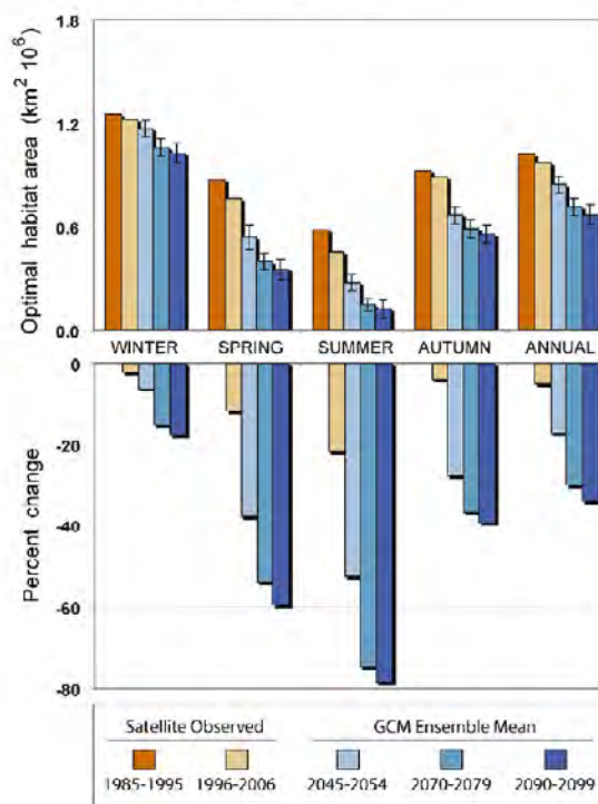
b) Alaska-Eurasia
