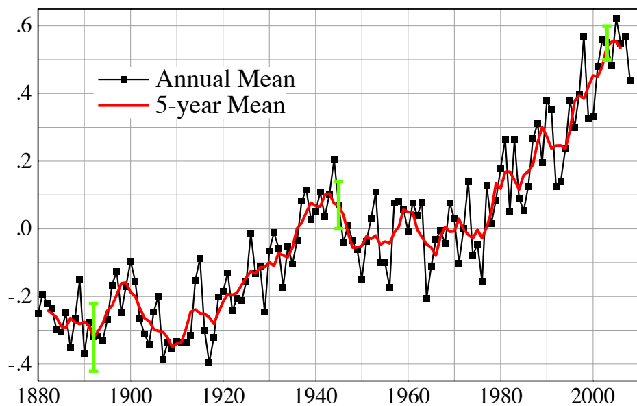
Global Land-Ocean Temperature Anomaly (°C)
