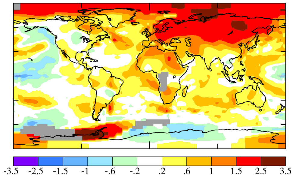
2008 Surface Temperature Anomaly (°C)
