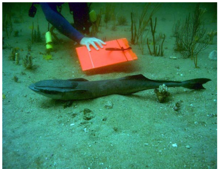
Image 27. Shark sucker.
