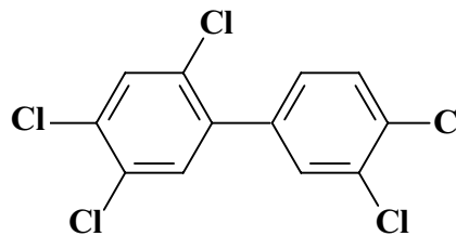
2,3',4,4',5-Pentachlorobiphenyl PCB 118
