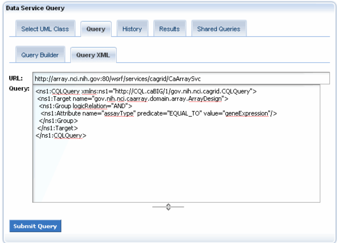
Figure 5-7. Query XML tab
