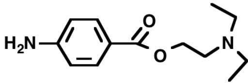
procaine
