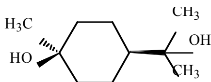
cis -Terpin
