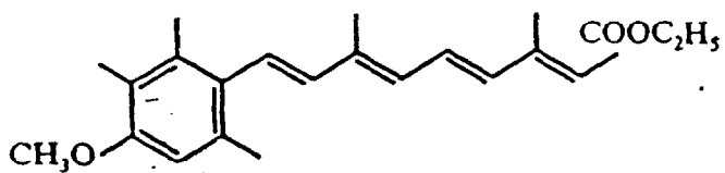
Etretinate
