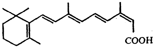
Isotretinoin
