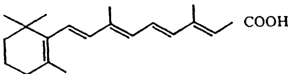
Tretinoin
