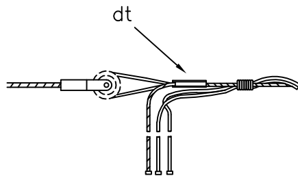
WEDGE TYPE
