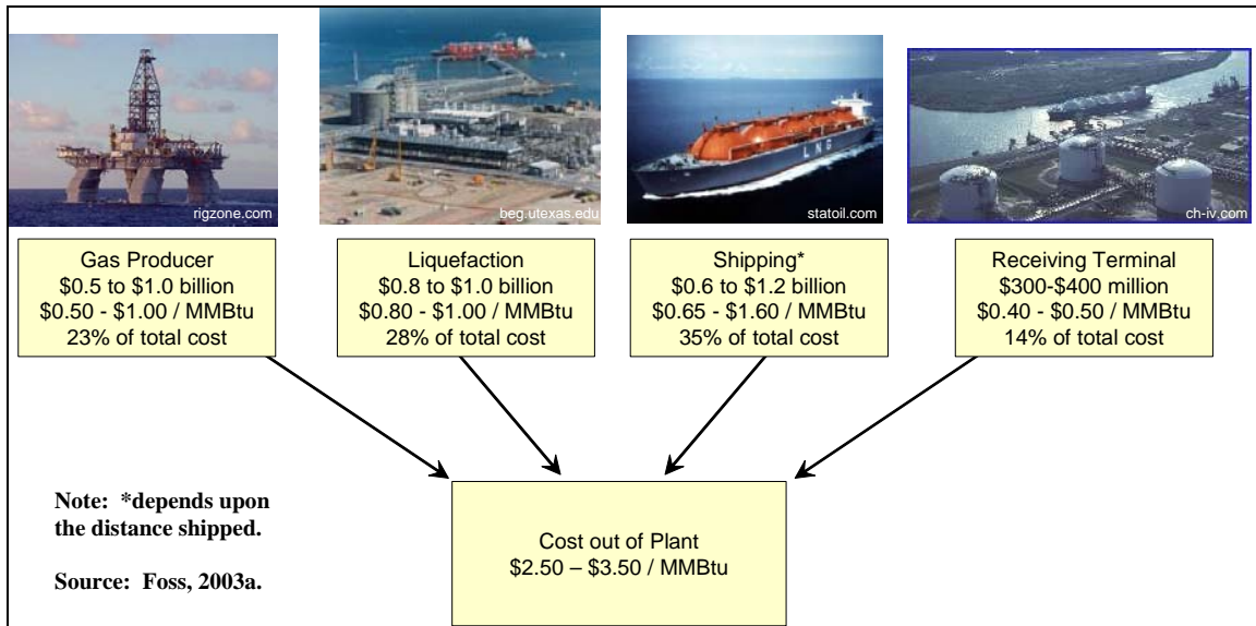
Figure 37. The LNG Value Chain.
