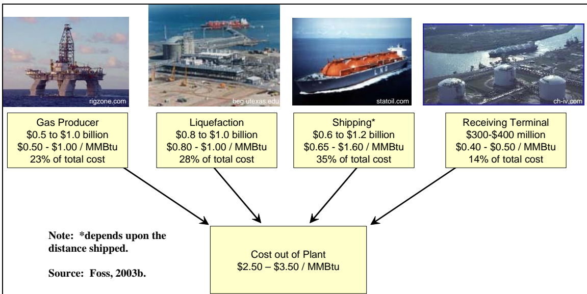
Figure ES.1. The LNG Value Chain.
