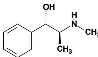
d -Pseudoephedrine
