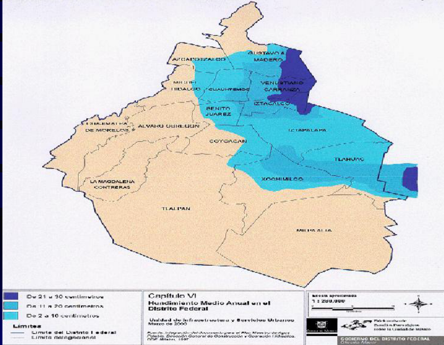
Hundimiento Medio Anual en el Distrito Federal
