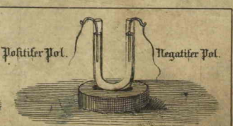
Zerlegung des Salzes durch die Electricität. Die Säure bezieht sich an den positiven, die Base an den negativen Pol.
