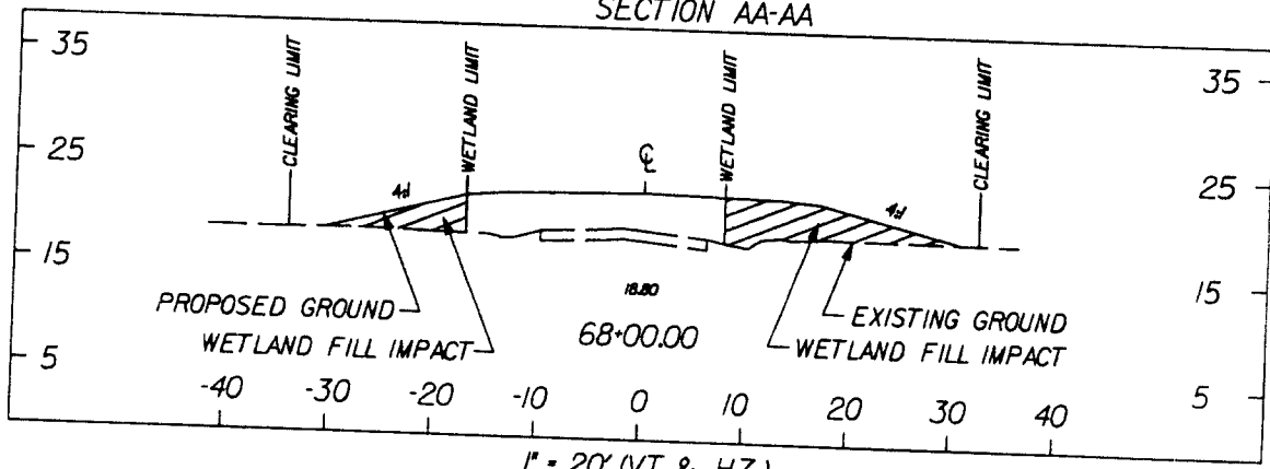
1" = 20' (VT. & HZ.)
