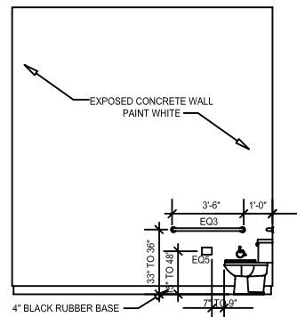
104 RESTROOM SCALE: 3/8" = 1'-0"
