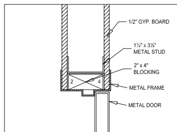
A JAMB
