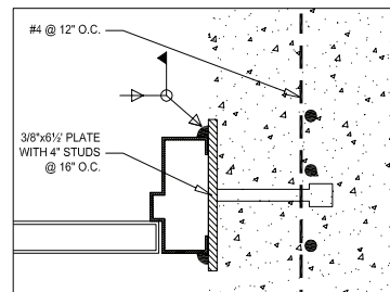
B JAMB
