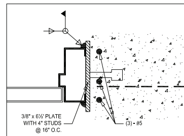
C JAMB
