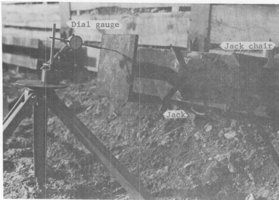
b) Bar tendon.
