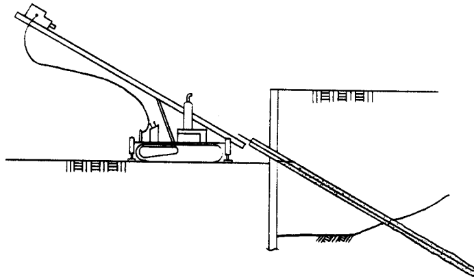
d) Insert the tendon.
