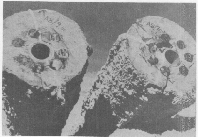
b) One inch tube à manchette tieback (courtesy Karl Bauer)
